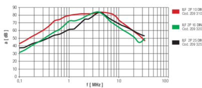
Curve caratteristiche di attenuazione asimmetrica
