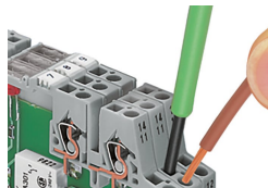
Connessione conduttore
