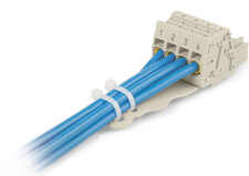
Piastrina antistrappo, per cablaggio in fabbrica Connettore femmina per 1 conduttore, 4 poli, passo pin 7,62 mm, grigio chiaro (831-3104/135-000)
