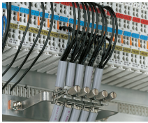
Barra collettiva in rame forma U 10 x 3 mm
