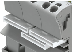
Collegamento a ponte agevole impiegando ponticelli orizzontali
