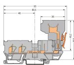
Morsetto di base
