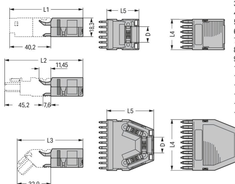
Dimensioni per gli alloggiamenti antistrappo
