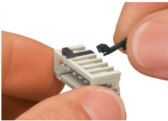
Codifica di un connettore maschio: le spine di codifica vengono innestate.
