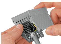
Custodia antistrappo mostrata con un connettore maschio dotato di CAGE CLAMP®
