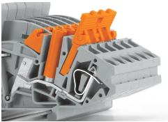
Ponticello con dispositivo di sicurezza Ponticello con dispositivo di sicurezza sollevato
