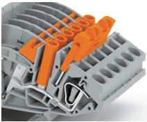
Ponticello con dispositivo di sicurezza Ponticello in posizione totalmente pre- serrata
