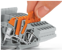
Ponticello con dispositivo di sicurezza Rimozione di un ponticello tramite dispo- sitivo di sicurezza.
