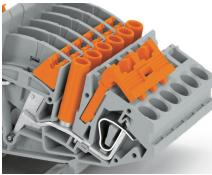
Ponticello con dispositivo di sicurezza Morsetti sezionatori azionabili longitudi- nalmente con ponticello integrato, inclu- so dispositivo di sicurezza
