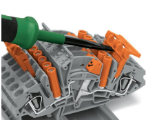
Ponticello con dispositivo di sicurezza Rimuovere il ponticello con l'utensile.
