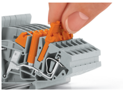
Ponticello con dispositivo di sicurezza Rimozione di un ponticello tramite dispo- sitivo di sicurezza.
