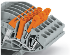
Ponticello con dispositivo di sicurezza Ponticello in posizione totalmente pre- serrata
