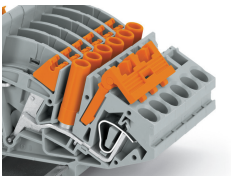
Ponticello con dispositivo di sicurezza Morsetti sezionatori azionabili longitudi- nalmente con ponticello integrato, inclu- so dispositivo di sicurezza
