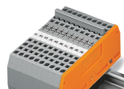
Collegamento a ponte con barre di ponticelli: Premere il ponticello a pettine in basso fino al completo inserimento.
