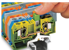
Il collegamento a ponte dei morsetti di terra e dei morsetti passanti è possibile in una sola direzione (tramite la parte posteriore del morsetto) usando ponticelli orizzontali. WAGO raccomanda l'impiego di ponticelli orizzontali giallo-verdi in aggiunta alla marcatura richiesta per questi tipi di morsetti.
