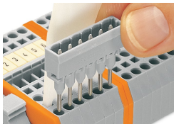
Inserimento di un conduttore maschio mediante utensile multipolo.
