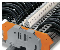
Marcatura dei morsetti con portaetichette doppio (209-128) Morsetti a marcatura laterale
