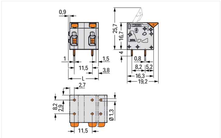
Misure in mm L = (n. poli - 1) x passo pin + 7,4 mm
