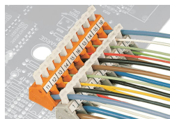
Sistemazione possibile dei conduttori con morsettiere sfasate (solo per serie 256).
