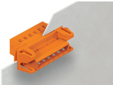
Connettore maschio con flange a scatto, per applicazioni passaparete del con spessore della piastra da 0,5 a 2,5 mm
