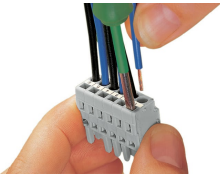
Inserimento del conduttore mediante cacciavite da 3,5 mm: azionamento di CAGE CLAMP® parallelamente rispetto all'ingresso del conduttore.
