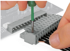
Inserimento di un conduttore mediante cacciavite da 3,5 mm: azionamento di CAGE CLAMP® perpendicolarmente rispetto all'ingresso del conduttore.
