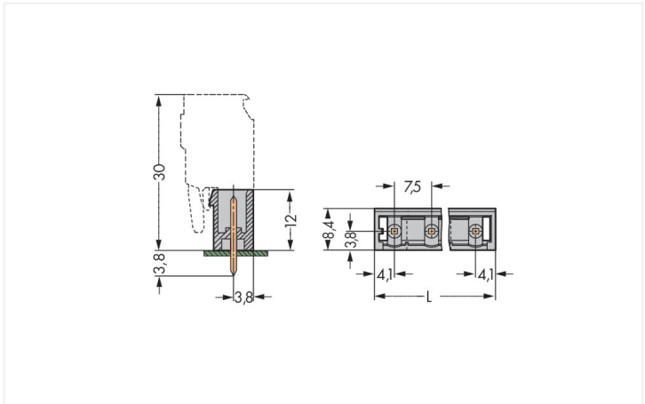
Misure in mm L = (n. \text{ poli} - 1) \times \text{passo pin} + 8,2 \text{ mm}
