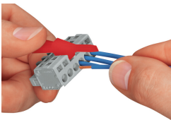
Terminazione del conduttore in perpendicolare all'azionamento CAGE CLAMP®
