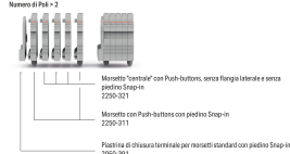
Esempio morsettiere a 5 poli con Push-button con piedini di fissaggio Strip-in
