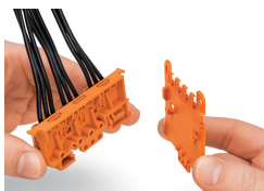
Fissaggio di una piastrina antistrappo (222-505) sul supporto di montaggio.
