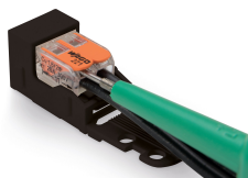
Collaudo di un connettore montato su un supporto mediante test slot.
