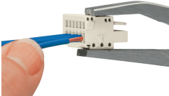
Inserimento di un conduttore mediante utensile di montaggio.
