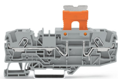
Morsetto di base (2006-401) con spina sezionatrice (2002-1661) in posizione di riposo
