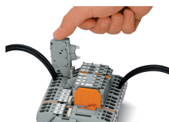
Morsetto sezionatore con fusibile con un portafusibile pivotante Ruotare il portafusibile fino alla posizione di bloccaggio.
