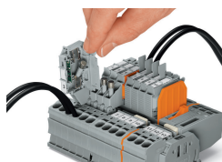
Morsetto sezionatore con fusibile con un portafusibile pivotante Sostituzione del fusibile: Aprire il coperchio per sostituire il fusibile
