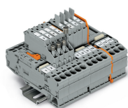
Porta fusibile pivotante con porta fusibile di riserva
