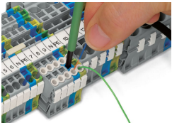
Collegamento dei conduttori: fermi- solante
