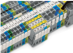
Fermisolante (2002-171) e copertura protettiva di avvertimento (2002-115)
