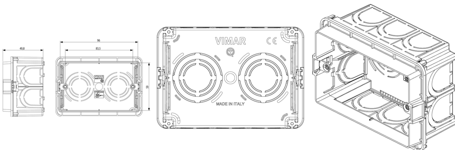
Vista ingombri
