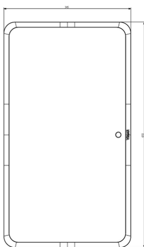
Vista ingombri
