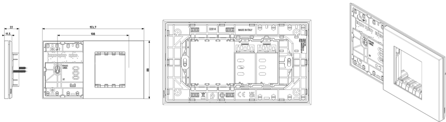
Vista ingombri
