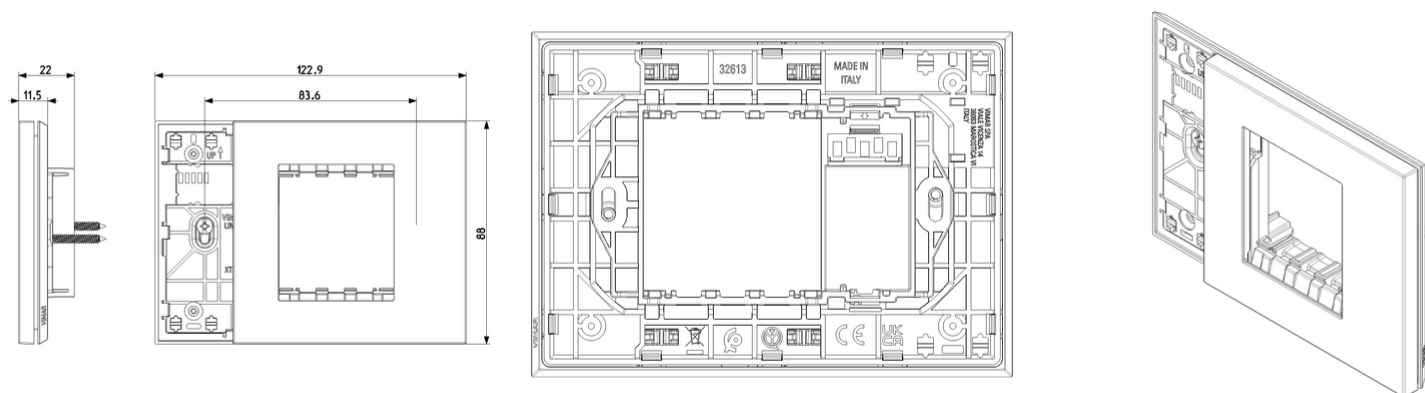
Vista ingombri
