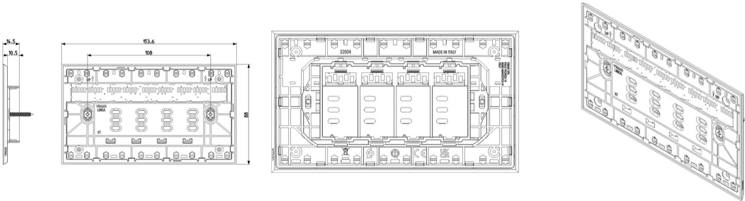
Vista ingombri
