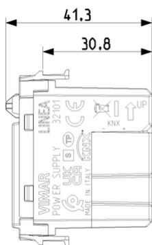
Vista ingombri
