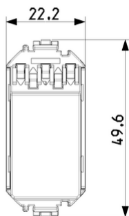
Vista ingombri
