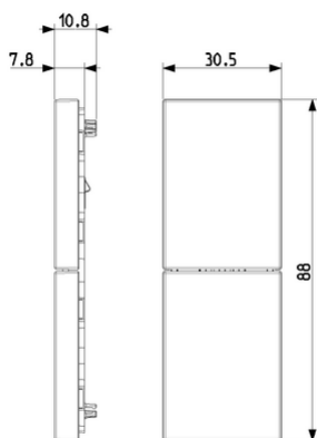
Vista ingombri
