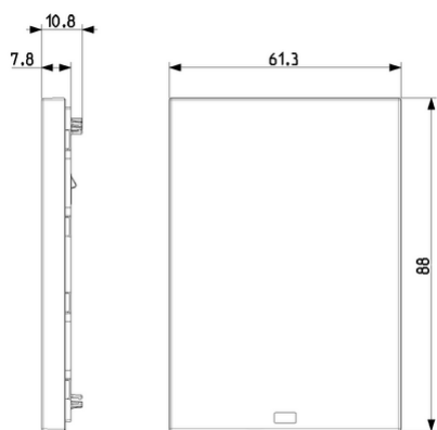
Vista ingombri
