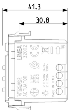
Vista ingombri
