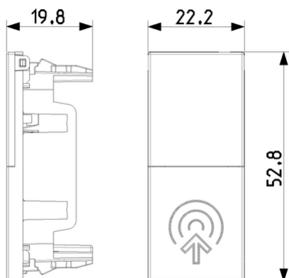
Vista ingombri
