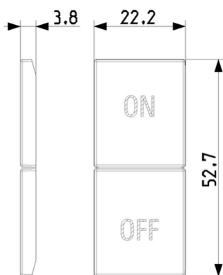
Vista ingombri
