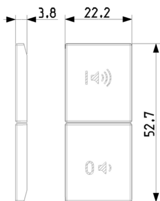
Vista ingombri
