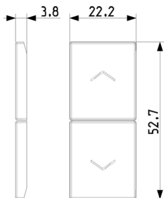
Vista ingombri
