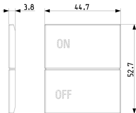
Vista ingombri
