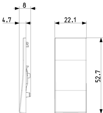
Vista ingombri
