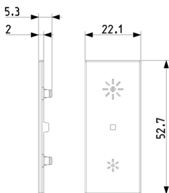
Vista ingombri
