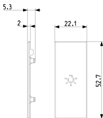
Vista ingombri
