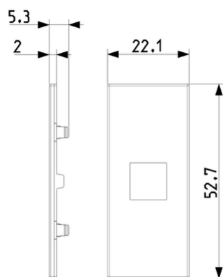
Vista ingombri
