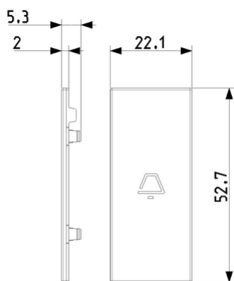
Vista ingombri
