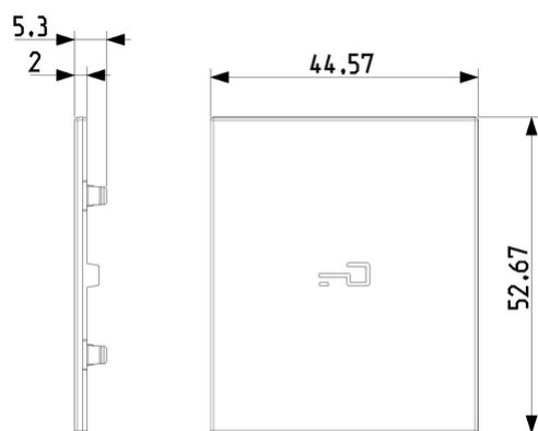
Vista ingombri
