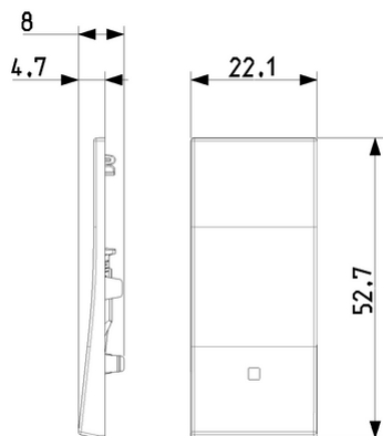
Vista ingombri
