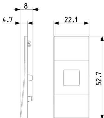
Vista ingombri
