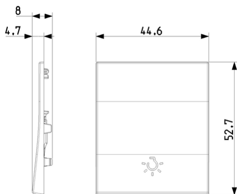
Vista ingombri
