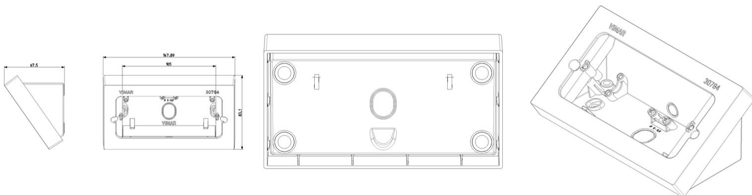
Vista ingombri
